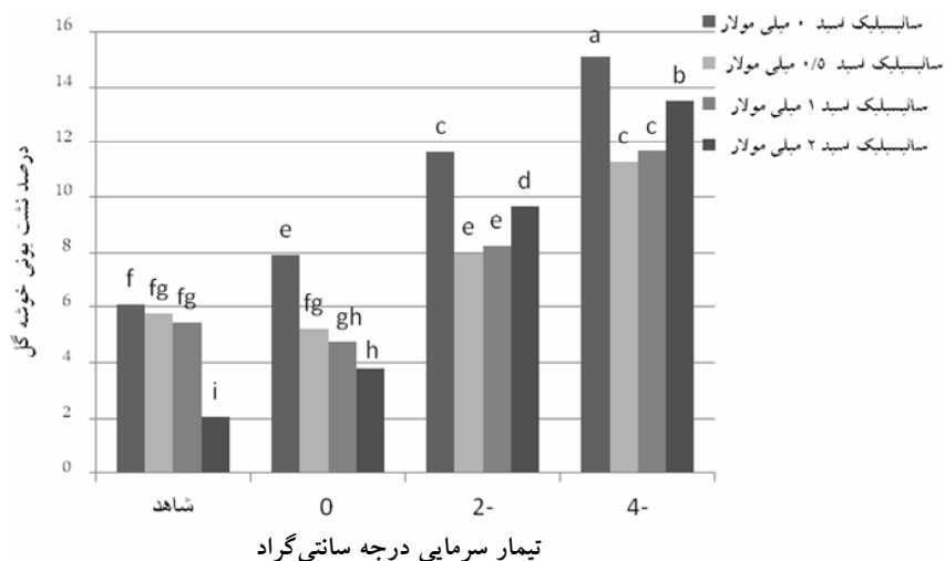
شکل ۳. اثر سالیسیلیک اسید بر درصد نشت یونی خوشه گل انگور رقم بیدانه سفید تحت تیمارهای سرمایی مختلف. حروف مشترک معرف نداشتن اختلاف معنی دار در سطح ۵ درصد است.
