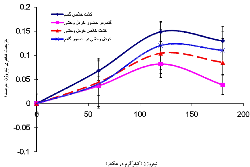
شکل ۱۴. واکنش بازیافت ظاهری نیتروژن به وسیله گندم و خردل وحشی به سطوح نیتروژن
