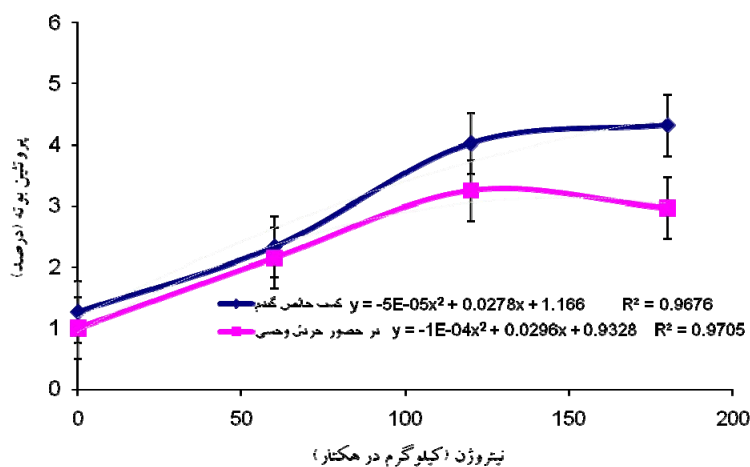
شکل ۱۰. واکنش پروتئین کل بوتۀ گندم به سطوح نیتروژن.
